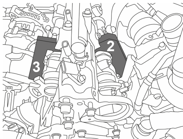
Outil de calage d'arbre à cames (3+2)
