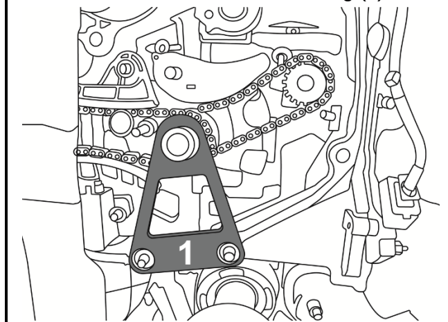
Kurbelwellen-Einstellwerkzeug (1)
