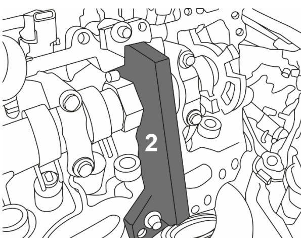
Nockenwellen-Einstellwerkzeug (2)
