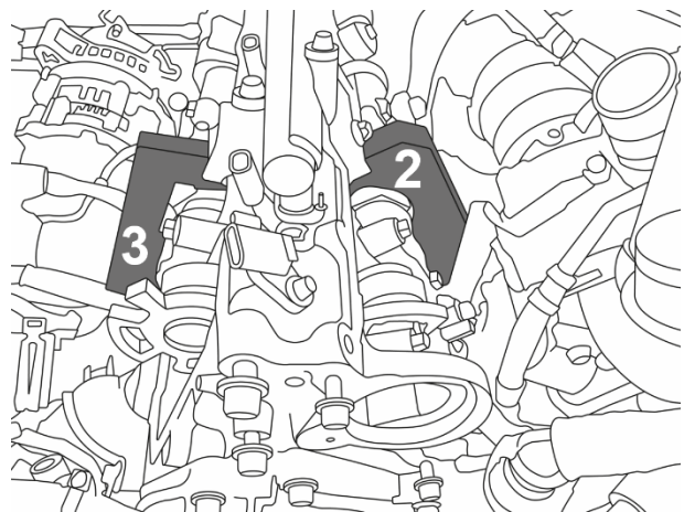
Herramienta de ajuste del árbol de levas (3+2)
