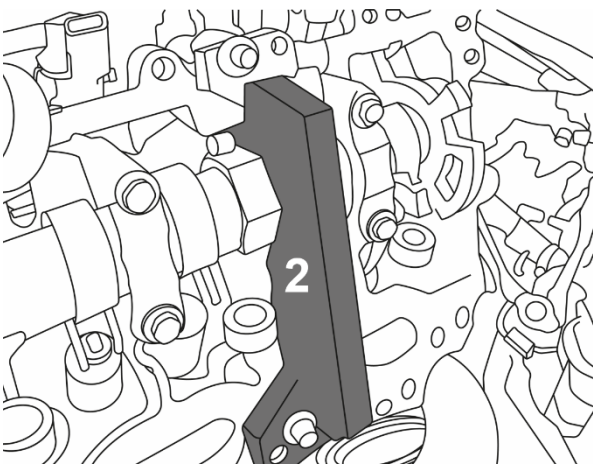
Herramienta de ajuste del árbol de levas (2)
