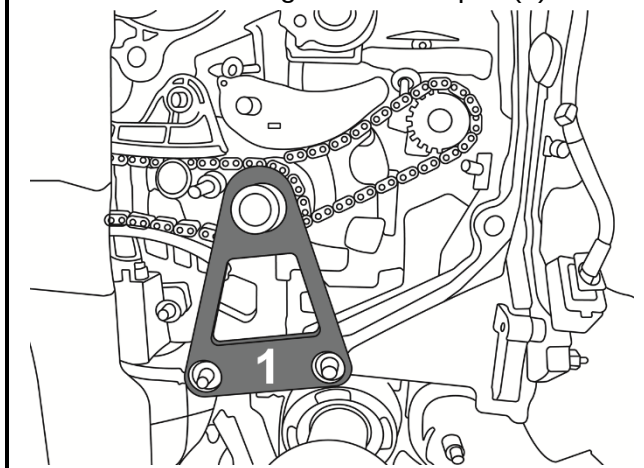
Outil de calage de vilebrequin (1)
