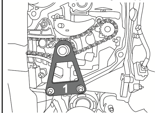
Herramienta de ajuste del cigüeñal (1)
