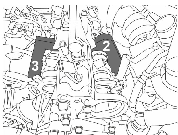
Nockenwellen-Einstellwerkzeug (3+2)
