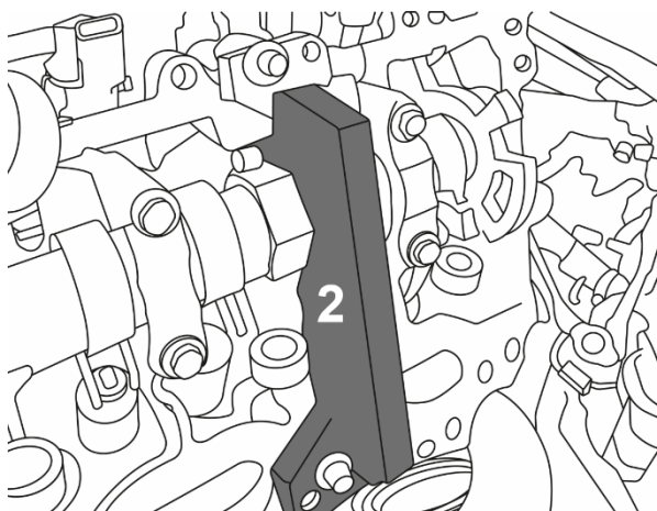
Outil de calage d'arbre à cames (2)
