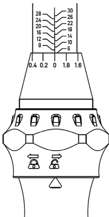
Geringster Wert 6 Nm
