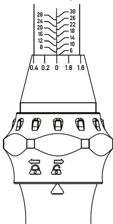
Valor más bajo 6 Nm
